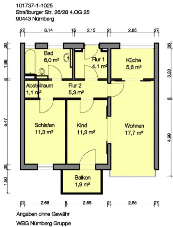
Grundriss
