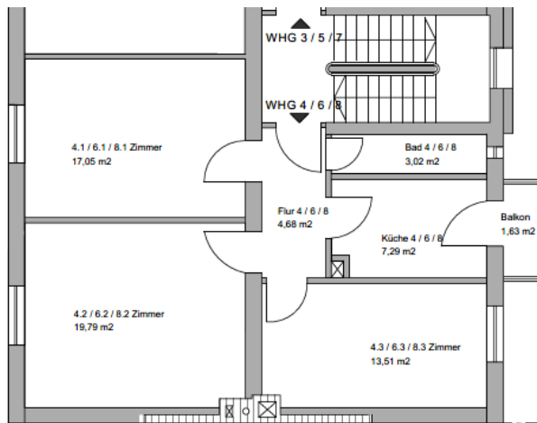
Grundriss
